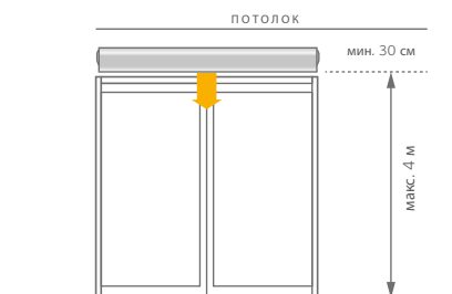
горизонтальный монтаж
